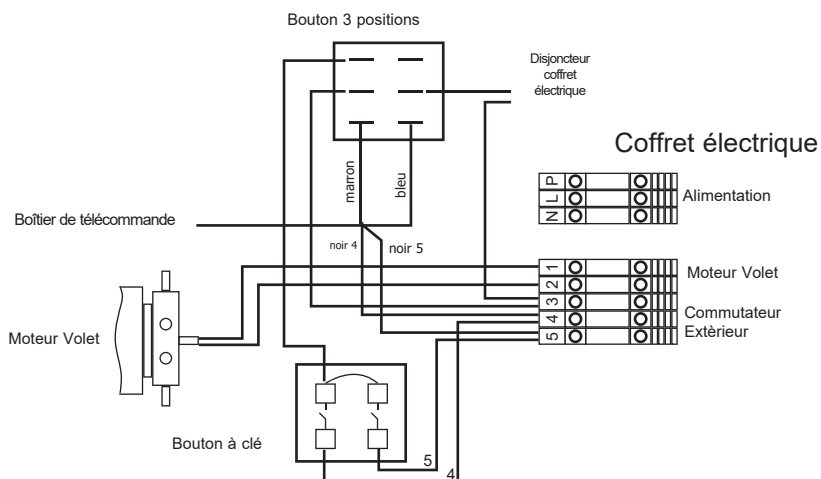
b - Borne motorisée "avec OPTION radicommande"
